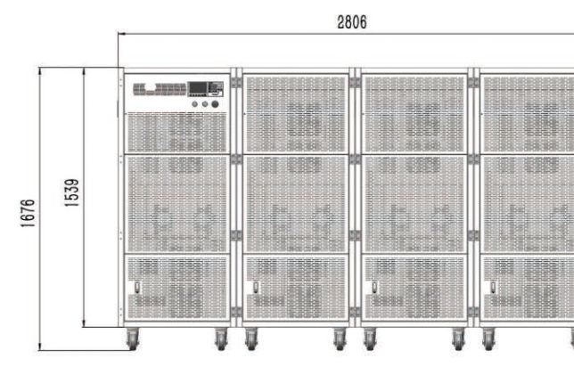
400KW机型
