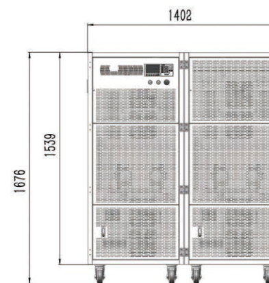
200KW机型
