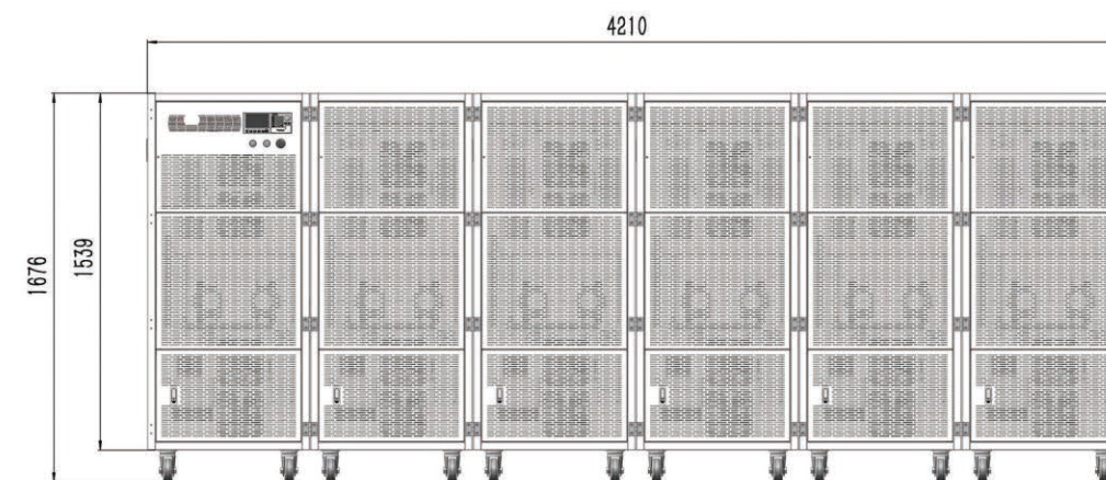
600KW机型
